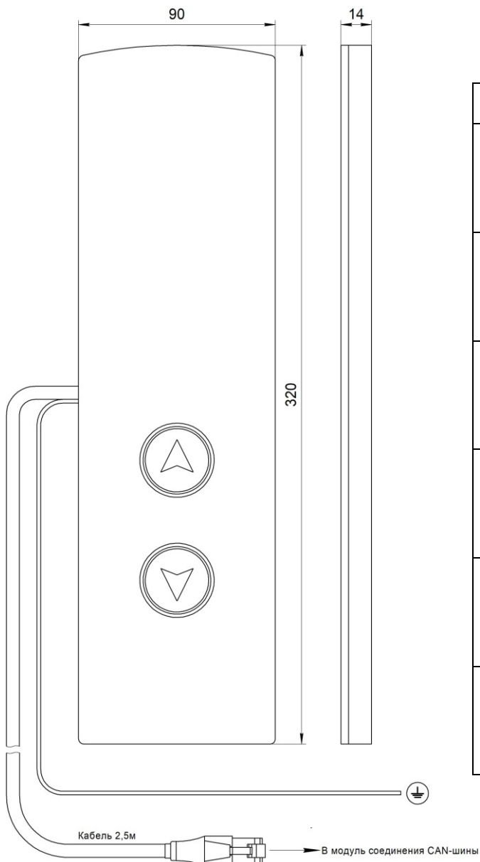
Рис.1 Внешний вид Вызывной пост ТОПАЗ (жгут RJ45) НШЕК.468381.206
